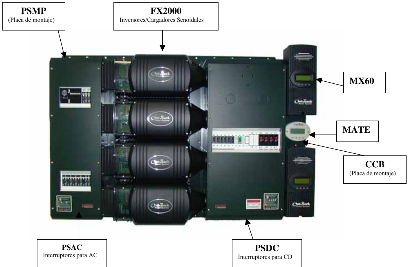
Fig.1 Una de las posibles formas de montar el MX60 junto con inversores FX de OutBack.
