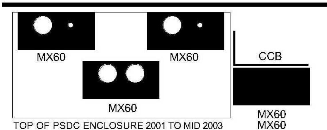
Fig.2 Alternativas para instalar los MX sobre el PSDC.
